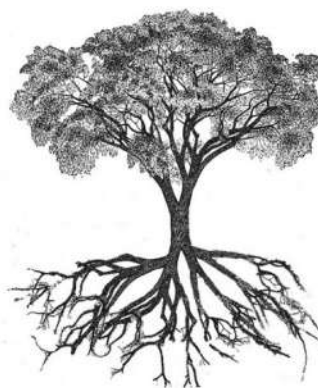
корень стержневой
